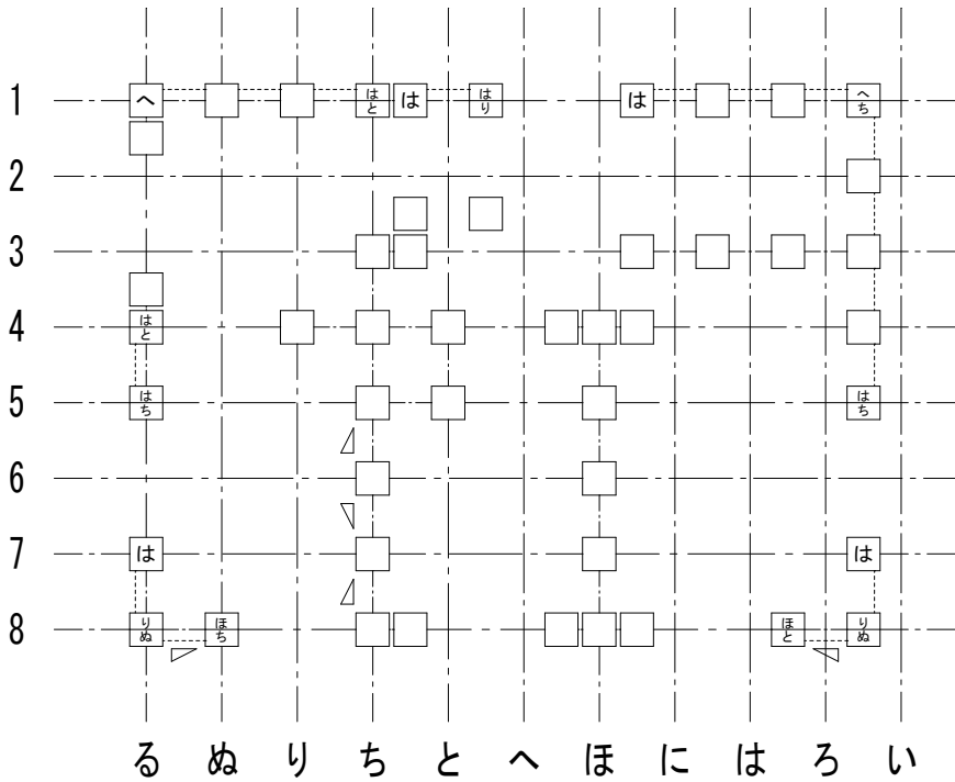
2 階柱壁伏図
