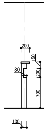
キッチン腰壁 断面
