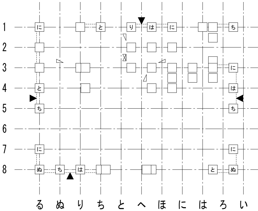
1 階柱壁伏図
